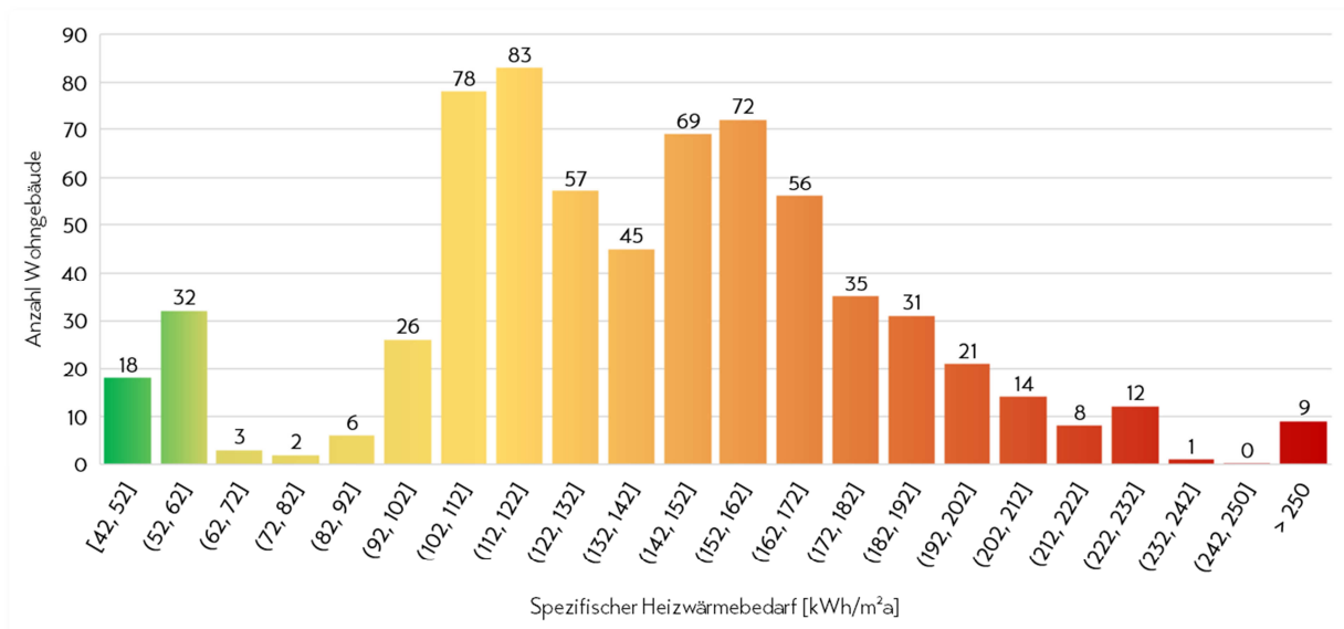
Abbildung 10: Energieeffizienz des Gebäudebestandes in der Gemeinde Bayerisch Gmain
