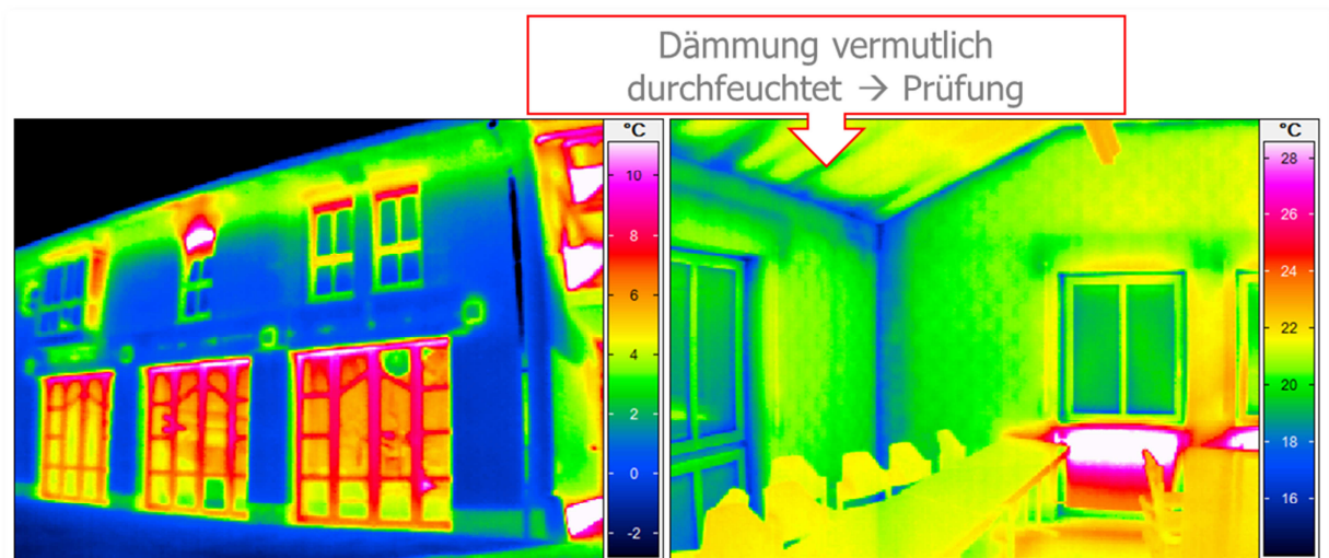
Abbildung 27: Thermografieaufnahme der Dachdämmung (FFW-Gebäude)
