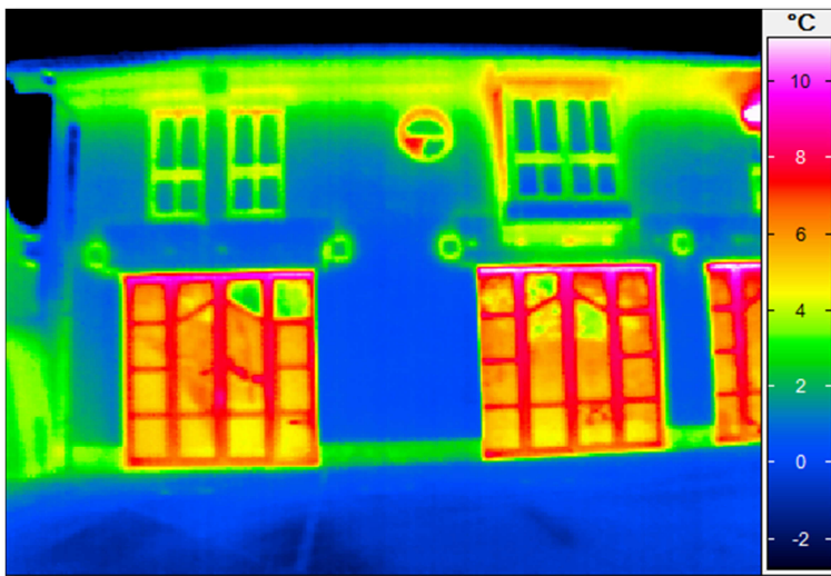
Abbildung 26: Thermografieaufnahme der Gebäudehülle (FFW-Gebäude)
