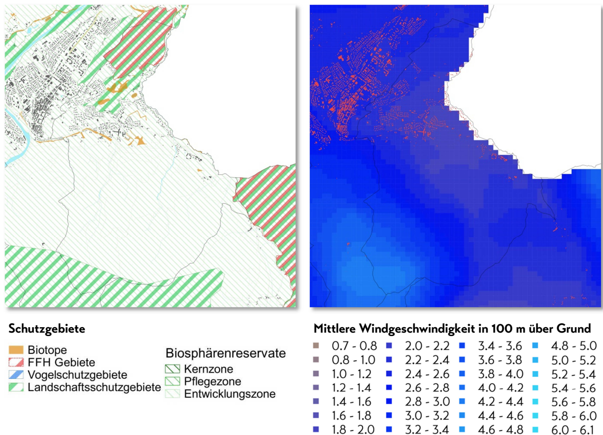
Abbildung 21: Schutzgebietskartierung (links) und mittlere Jahreswindgeschwindigkeit in 100 m ü. G. (rechts)
